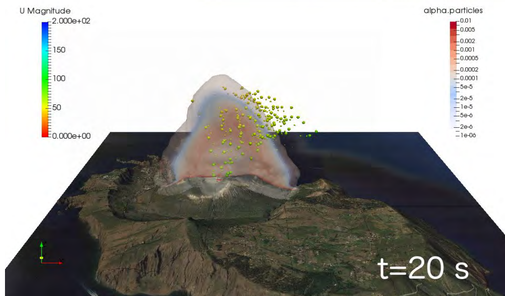
Simulazione numerica tridimensionale della formazione di correnti piroclastiche e della eiezione balistica durante l'eruzione idrotermale della Breccia di Commenda a Vulcano (isole Eolie, Italy) (immagine di Tomaso Esposti Ongaro, INGV - Sezione di Pisa).
