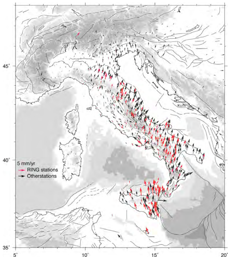
Campo di velocità orizzontale misurato dalla rete RING (Rete Integrata Nazionale GPS) sul territorio nazionale (freccie rosse) e da altre reti GPS (freccie nere), da Devoti et al. (2017).
